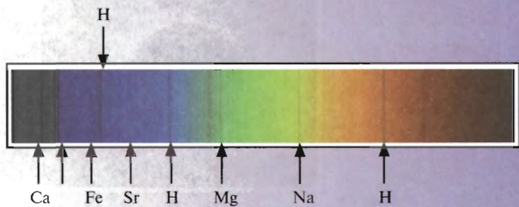
Рис. XIII. Солнечный спектр.
